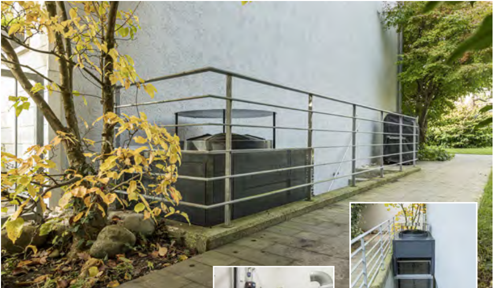
Schwabender Einbau der Ausseneinheit beim Kellereingang, Heizungskeller mit Heizungspeicher und Wärmepumpenboiler.
